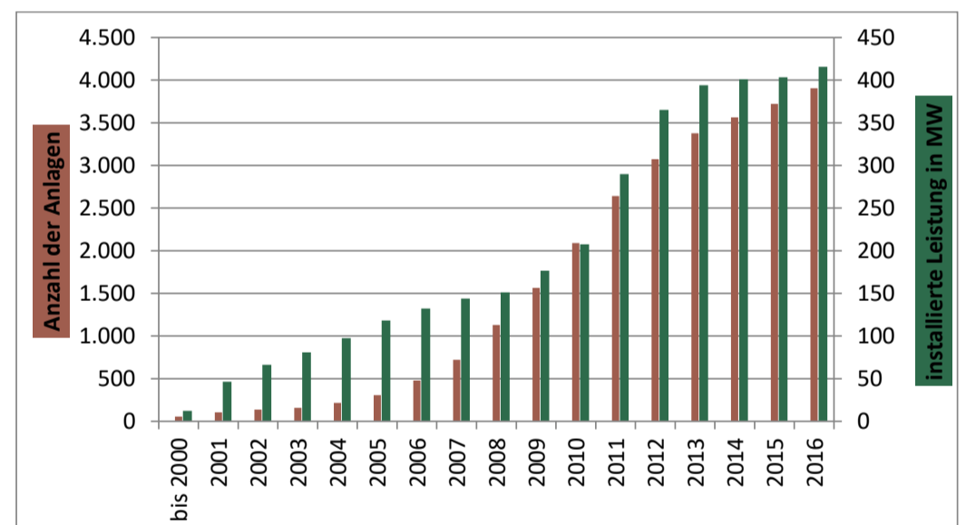
Entwicklung der Anlagenanzahl und der installierten Leistung zur Erzeugung von Strom aus regenerativen Energiequellen im Landkreis Bautzen von 2000 bis 2016
